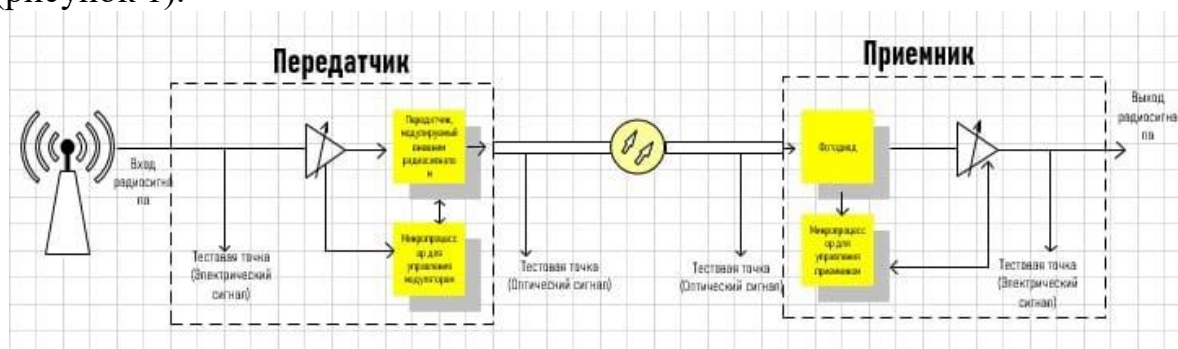
Рисунок 1 – Оптические компоненты
