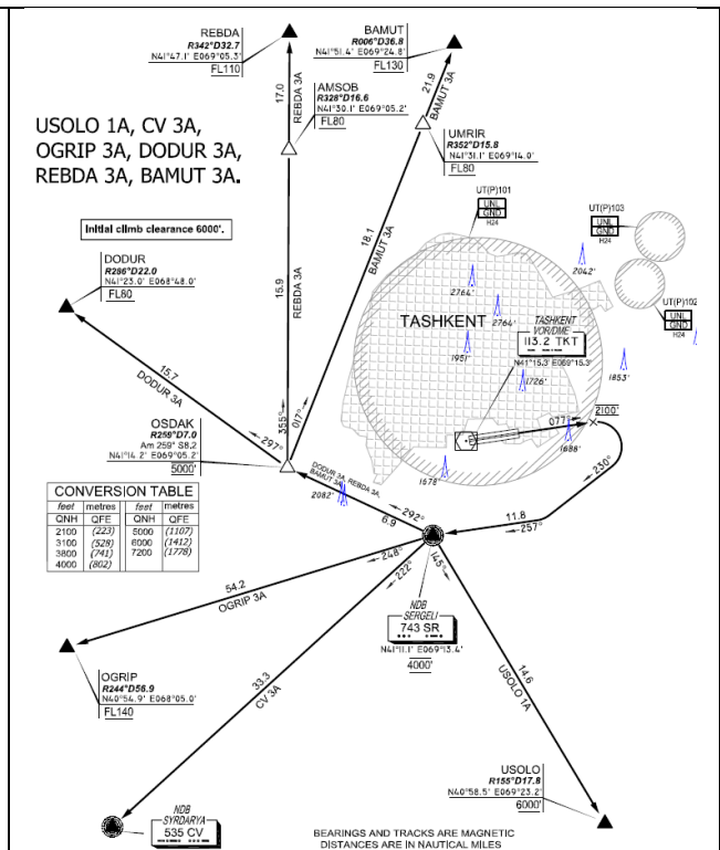
Рис. 1 б. Стандартные маршруты вылета SID UT TT RW08R/L
