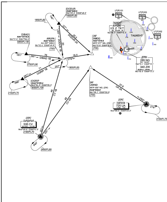
Рис. 1 а. Стандартные маршруты прибытия STAR UT TT RW08R/L
