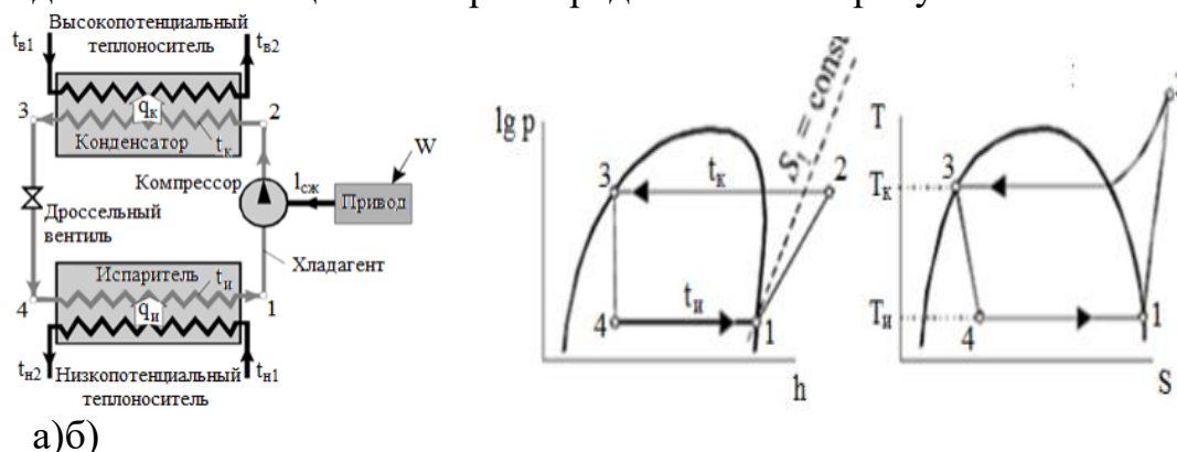
Рисунок 1 – Парокомпрессионный тепловой насос; а – принципиальная схема, б – термодинамический цикл
