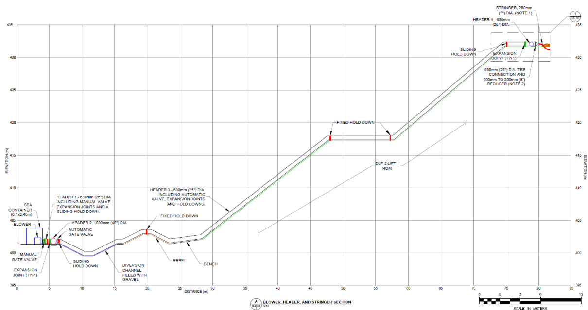
Рис.2 Общий вид системы аэрации ПКВ2
