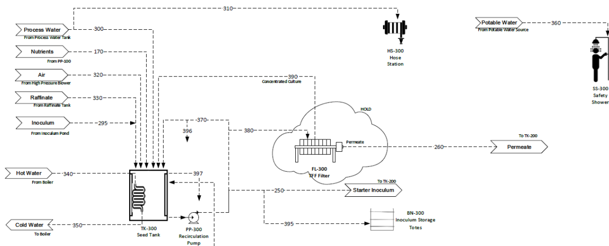
Рис.7 Технологическая схема участка начальной культуры (ТК-300 – семенной резервуар, в котором происходит смешивание питательных веществ, рафината и инокулята из пруда инокулята для получения начального инокулята)
