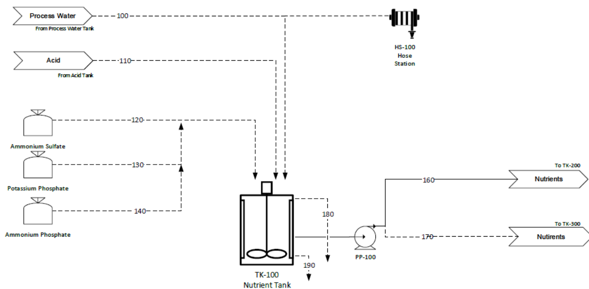
Рис.5 Технологическая схема участка реагентов (ТК-100 – резервуар для питательных веществ)
